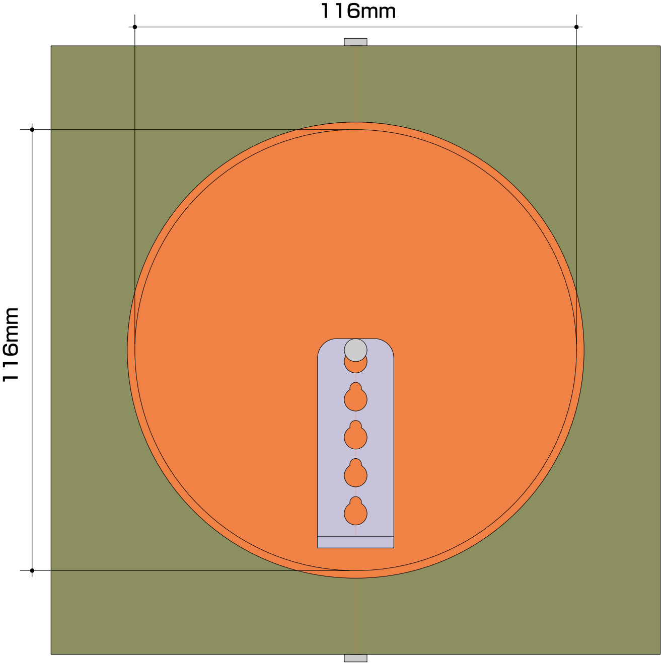
正面図
