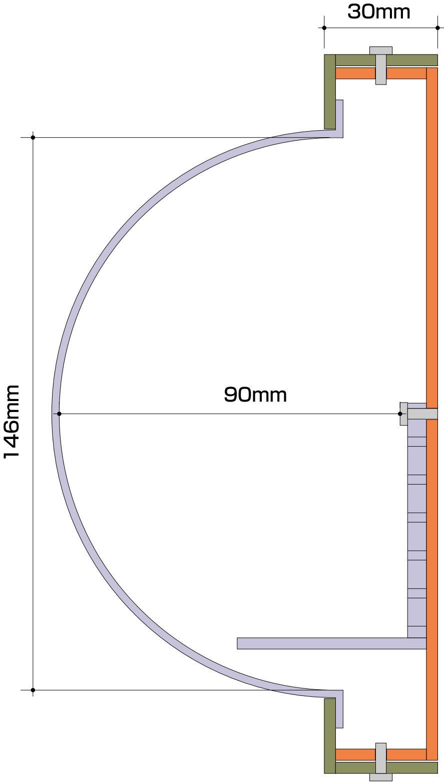
断面図
